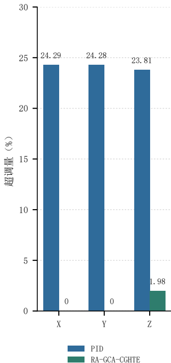
(a) 三轴阶跃超调
