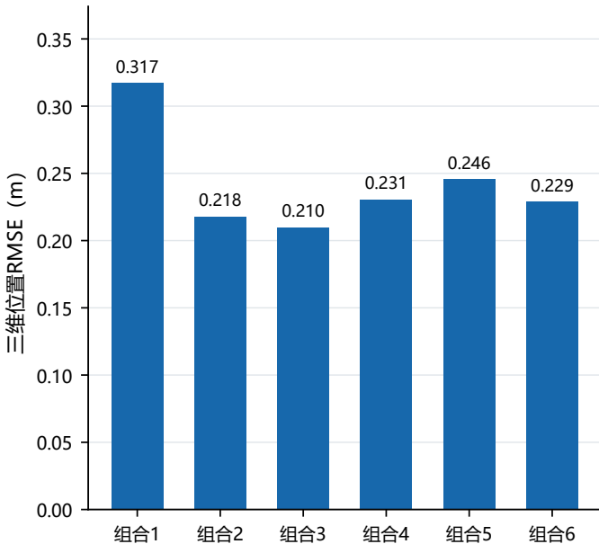
复合扰动下的跟踪误差
