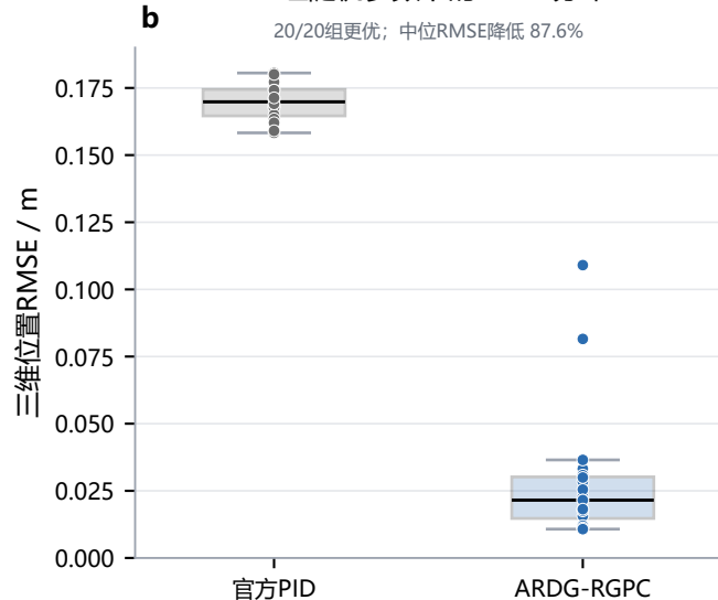
20组随机参数下的RMSE分布
