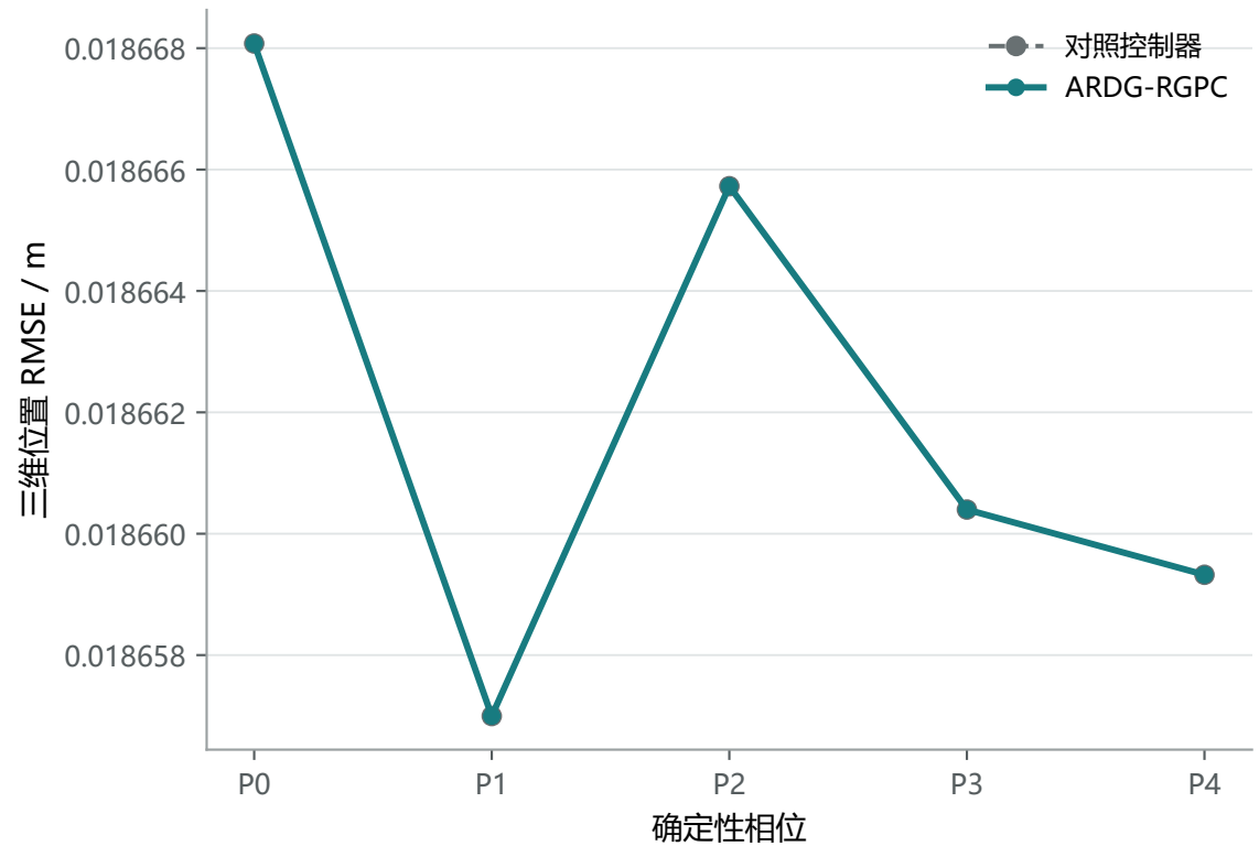
(b) 五相位传感器退化
