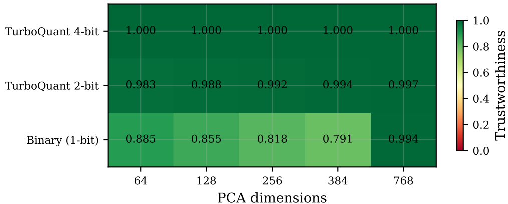
trec-covid — Trustworthiness (k=50)
