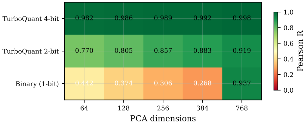
fiqa — Pearson r
