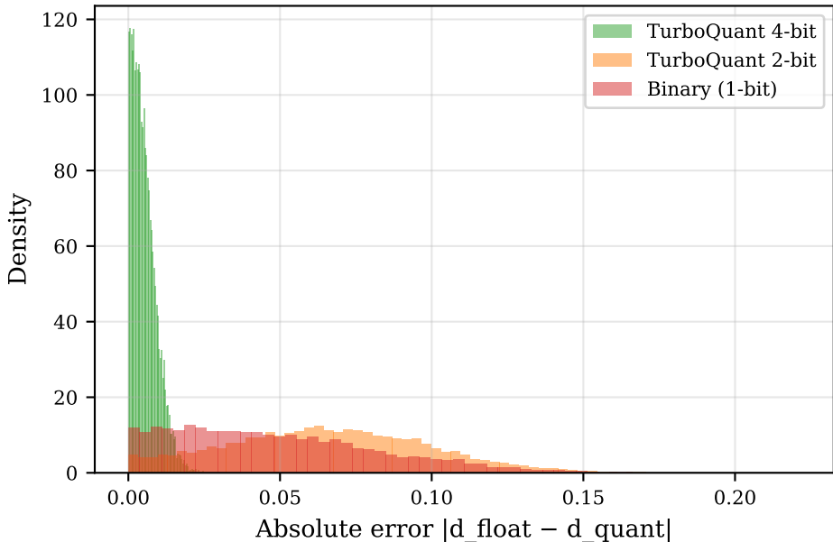
scifact (d=768)
