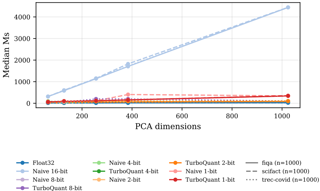
NumPy top k
