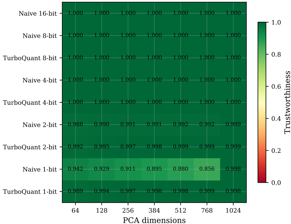
trec-covid — Trustworthiness (k=10)
