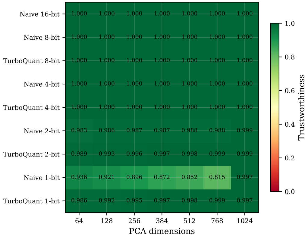
scifact — Trustworthiness (k=20)
