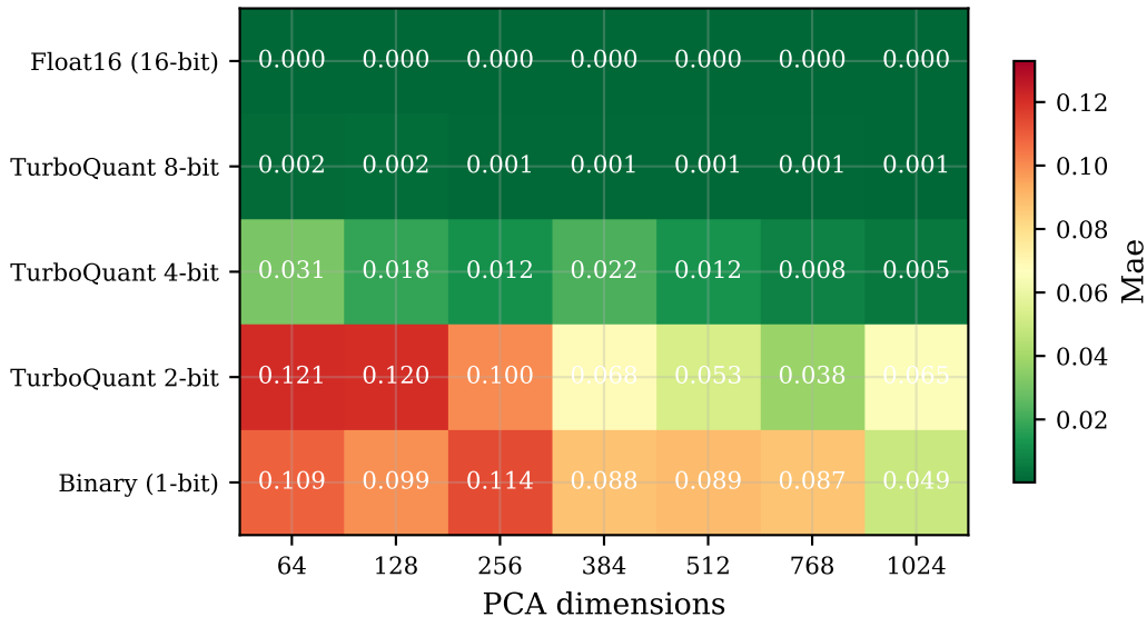
scifact — MAE
