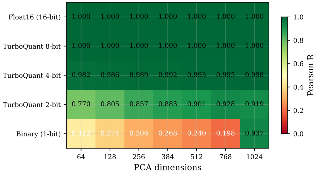
fiqa — Pearson r
