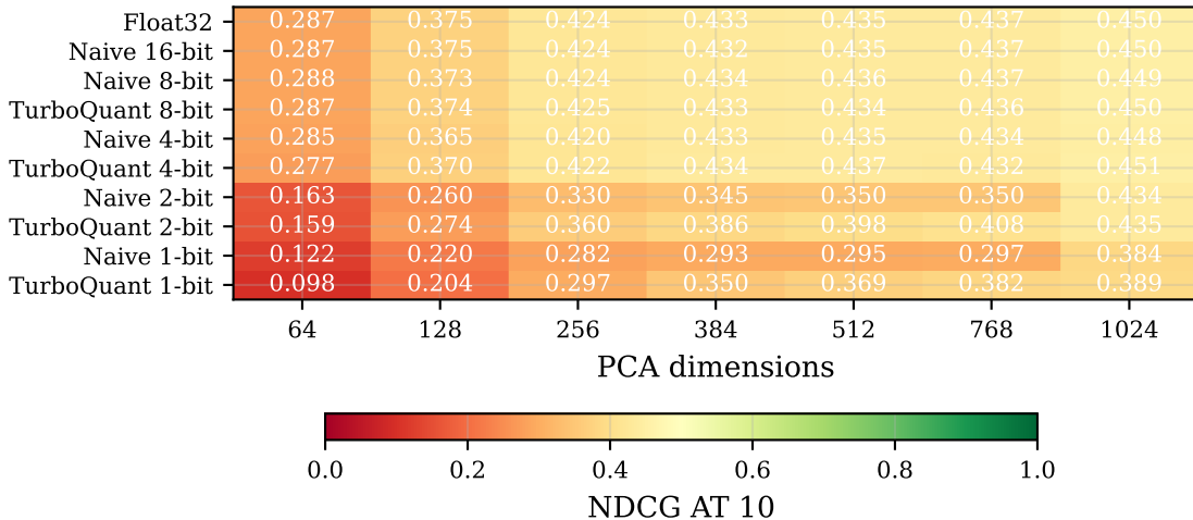
fiqa - NDCG@10
