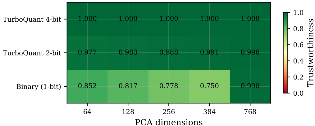
trec-covid — Trustworthiness (k=100)
