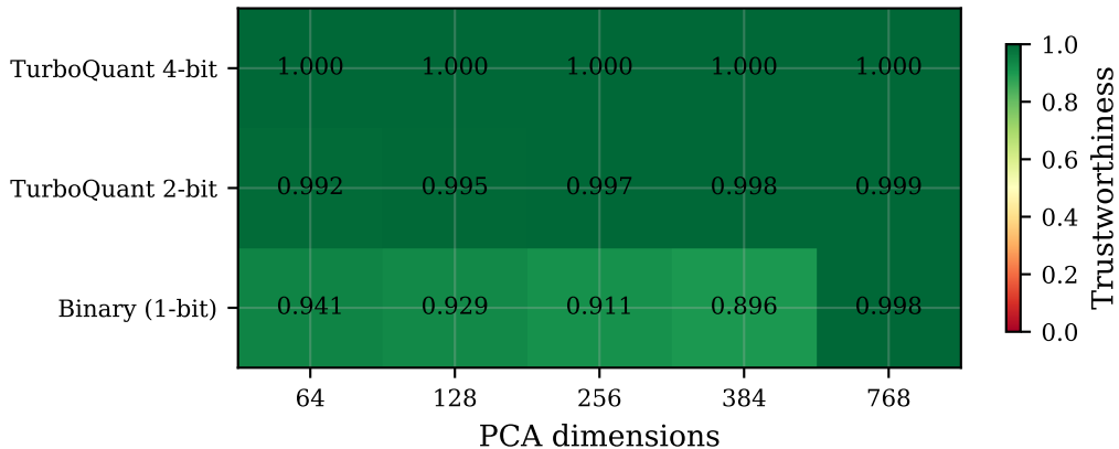
trec-covid — Trustworthiness (k=10)
