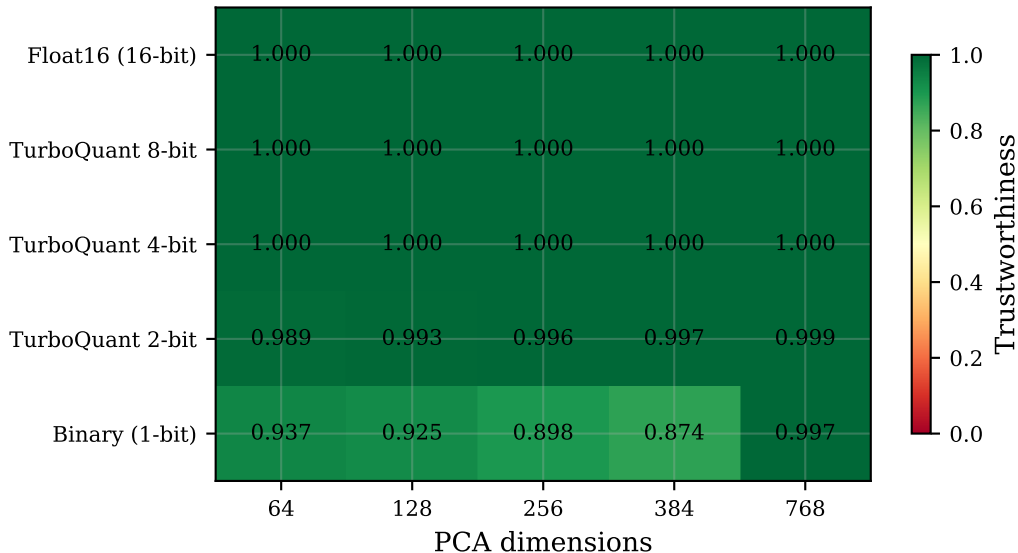
scifact — Trustworthiness (k=20)
