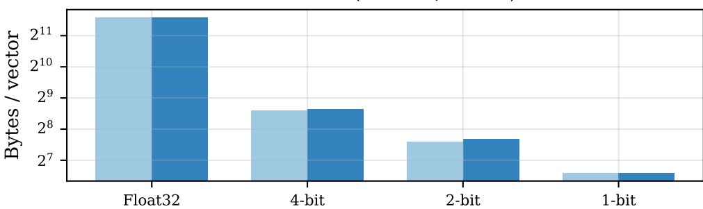
trec-covid (n=1000, d=768)
