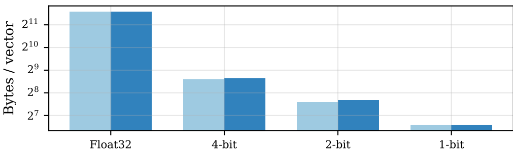
trec-covid (n=1000, d=64)
