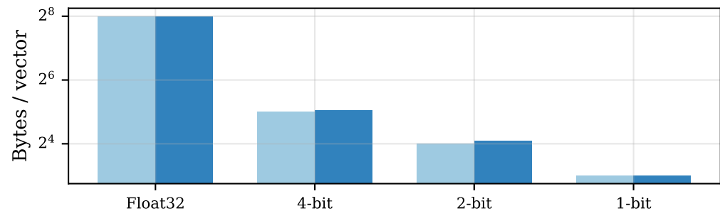
scifact (n=1000, d=768)
