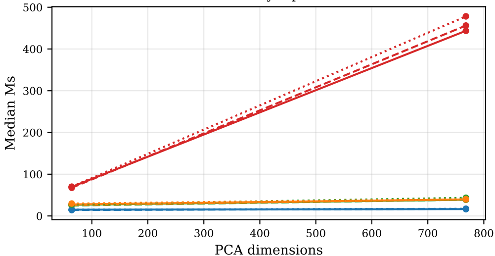
NumPy top k
