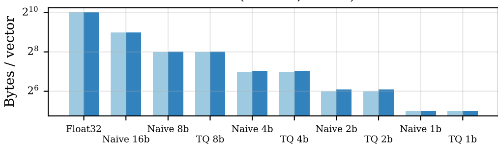
scifact (n=1000, d=384)
