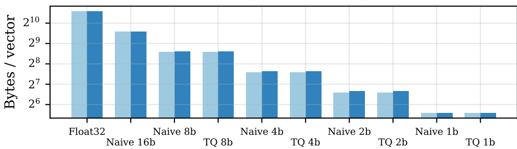
scifact (n=1000, d=768)
