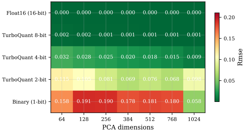
fiqa — RMSE
