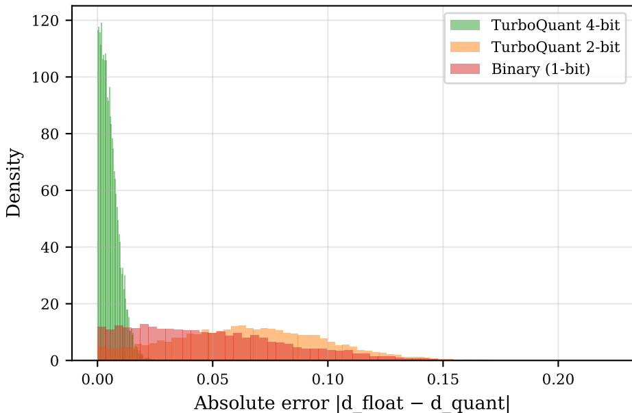
scifact (d=1024)
