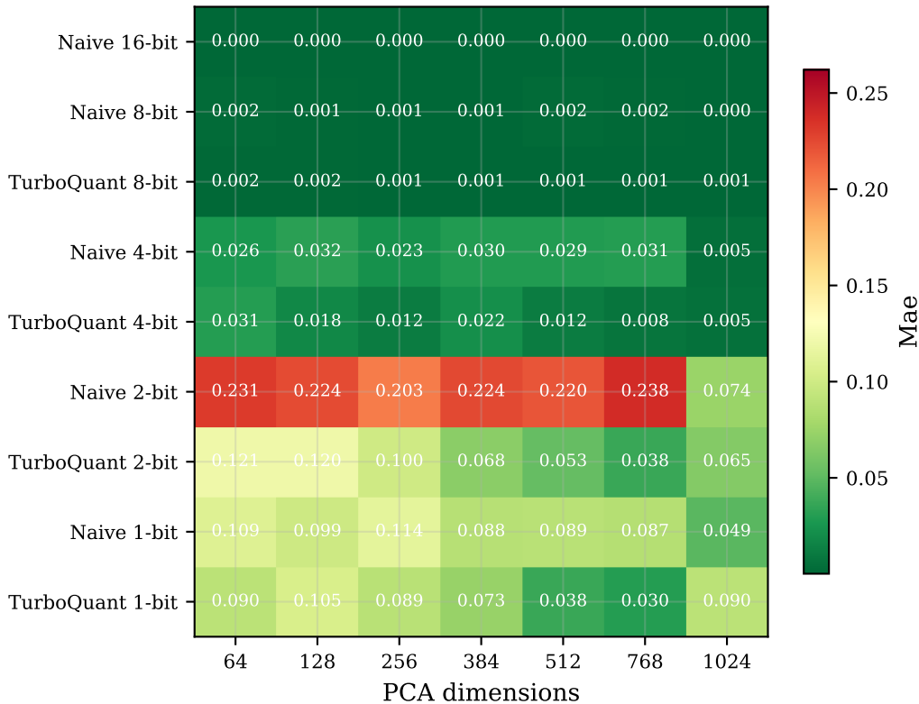
scifact — MAE
