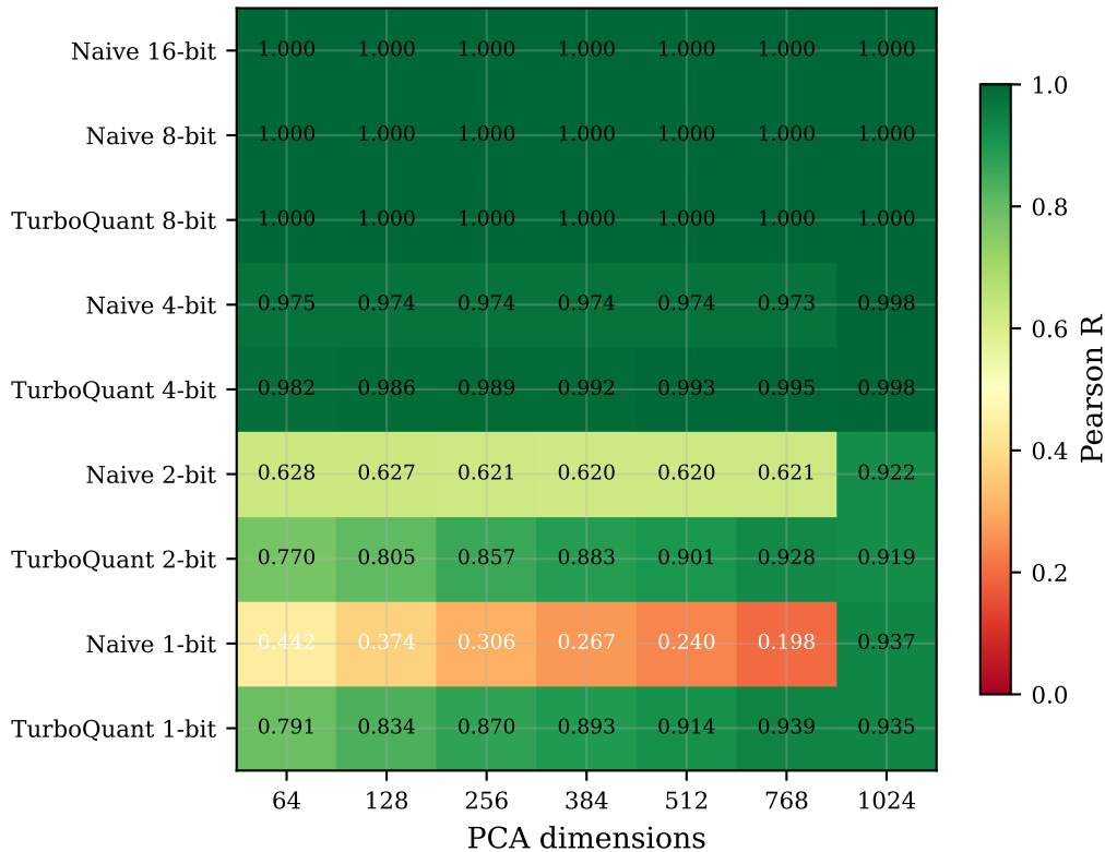
fiqa — Pearson r
