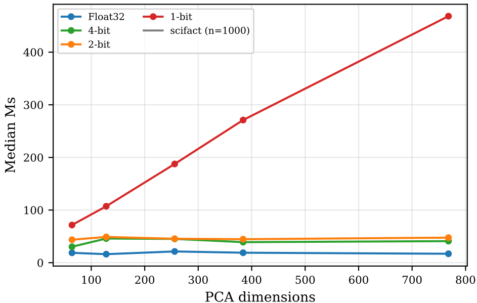
NumPy top k
