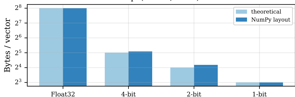
fiqa (n=1000, d=64)
