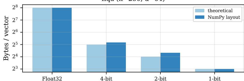
fiqa (n=500, d=64)
