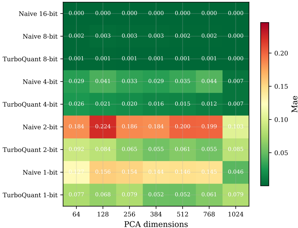
fiqa — MAE
