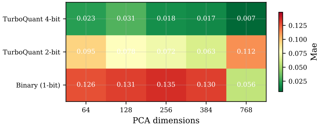
trec-covid — MAE
