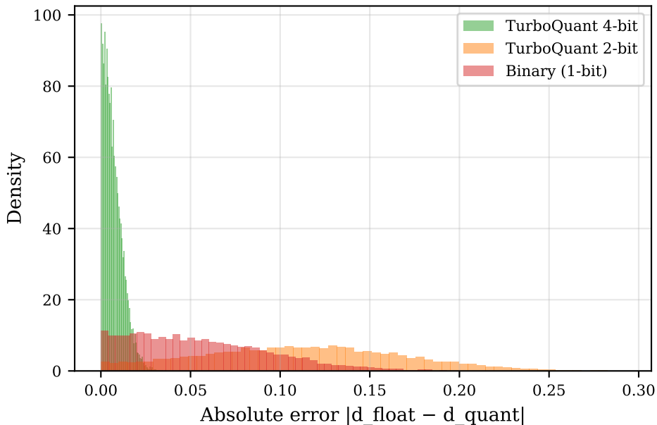
trec-covid (d=768)
