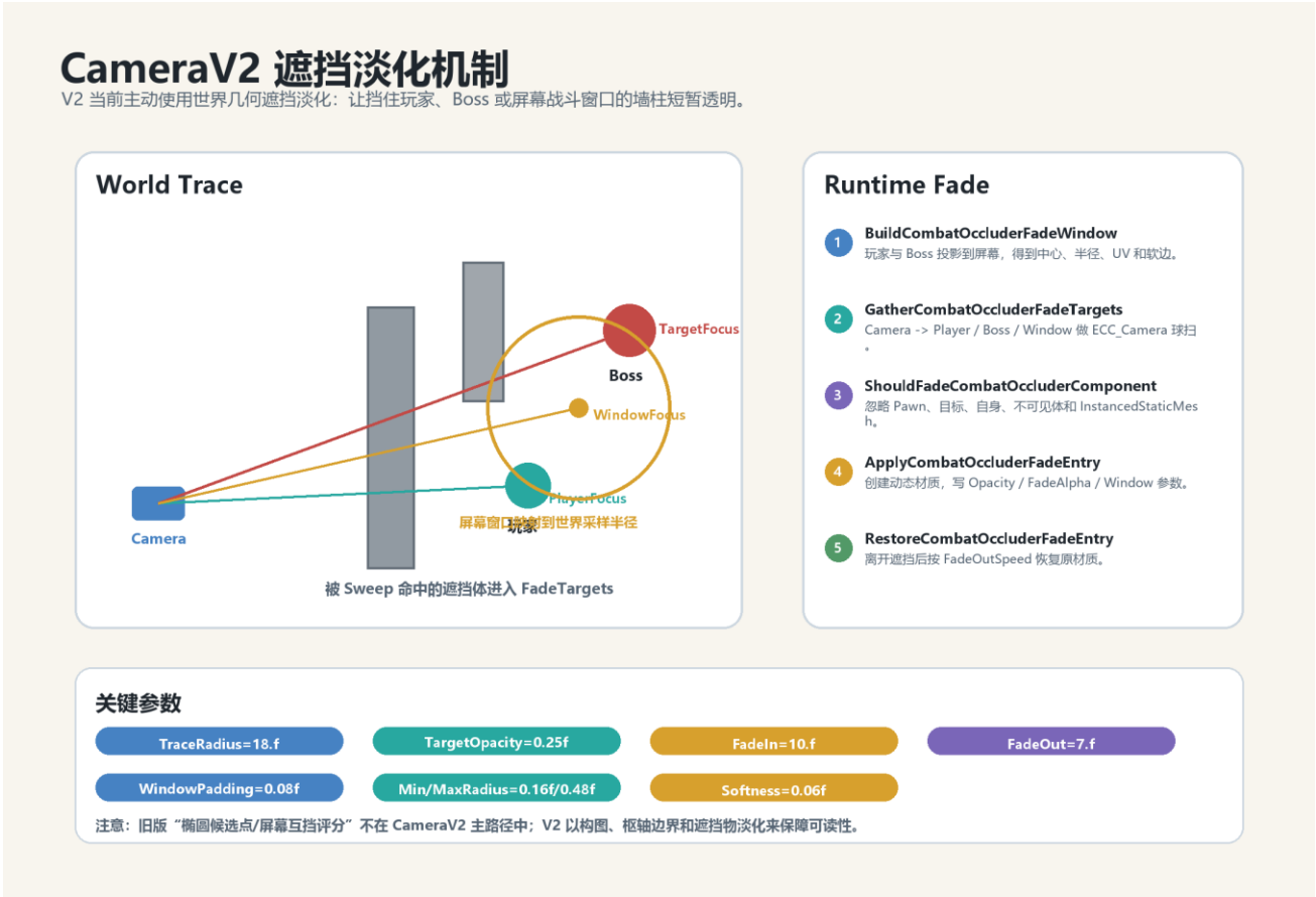
图 3C-7 CameraV2 世界遮挡淡化：球扫、屏幕窗口与动态材质
