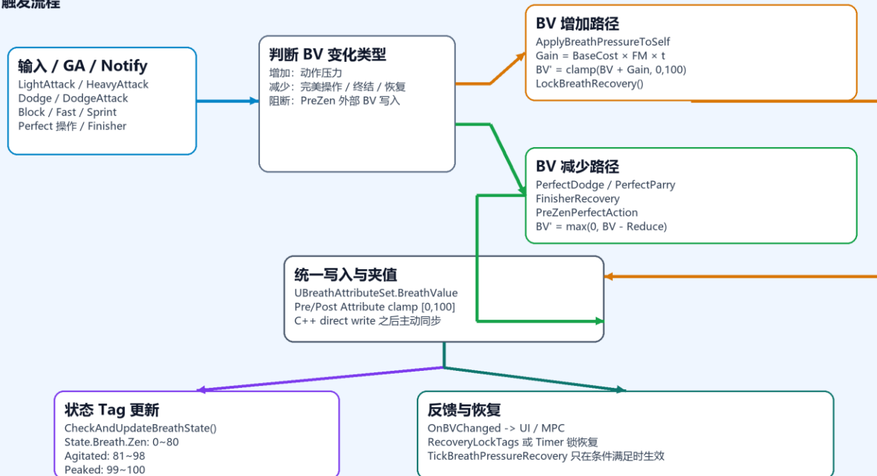
图 4-2A 呼吸值触发逻辑：行为输入、BV 写入、状态 Tag 与恢复锁
