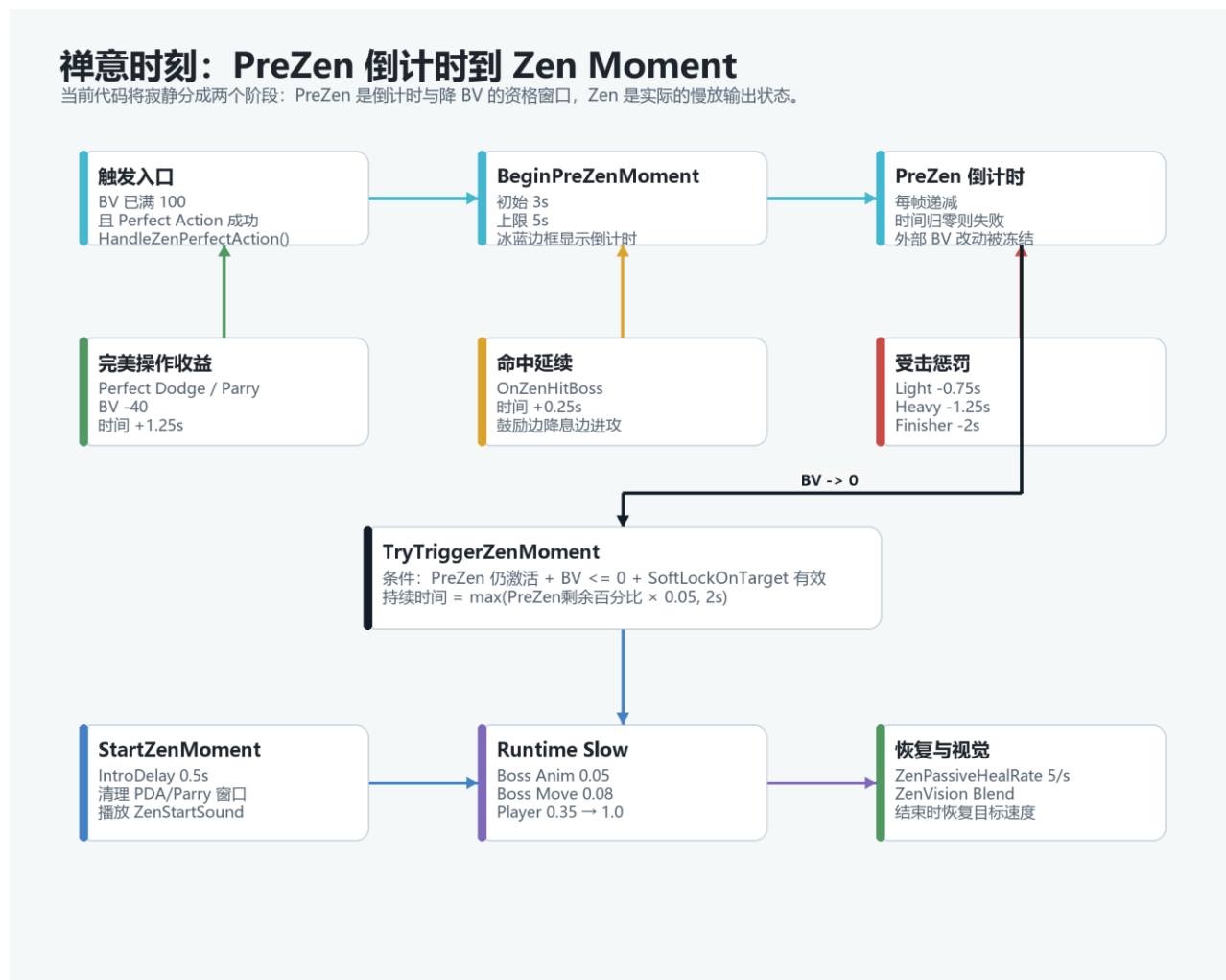
图 4-5 禅意时刻流程：PreZen 倒计时、BV 归零与 Zen Moment 慢放
