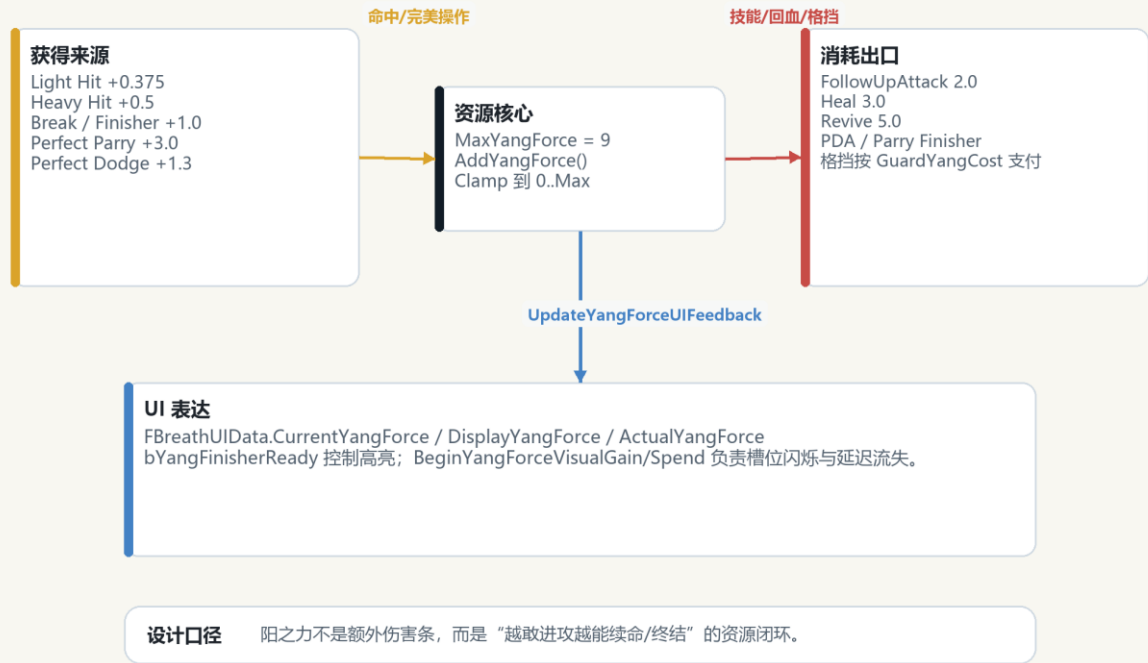
图 4-4 阳之力资源闭环：获得、存储、消耗与 UI 槽位反馈
