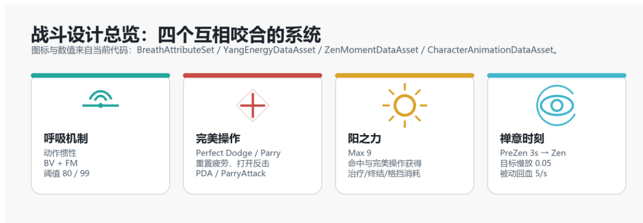
图 4-1 战斗设计四系统总览：呼吸、完美操作、阳之力与禅意时刻
