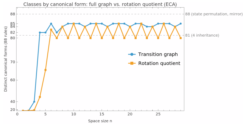
Fig. 3: Número de formas canónicas distintas entre las 88 reglas representantes con el grafo de transición completo y con el grafo cociente por traslaciones, para n = 1, \dots, 29 (eje vertical en escala cúbica).
