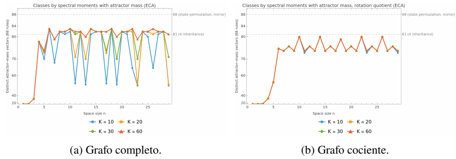
Fig. 7: Número de vectores de momentos espectrales con masa de atractor distintos entre las 88 reglas representantes para n = 1, \dots, 29 y K = 10, 20, 30, 60 .
