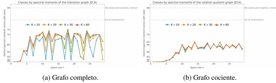
Fig. 5: Número de vectores de momentos espectrales distintos entre las 88 reglas representantes para n = 1, \dots, 29 y K = 10, 20, 30, 60 .
