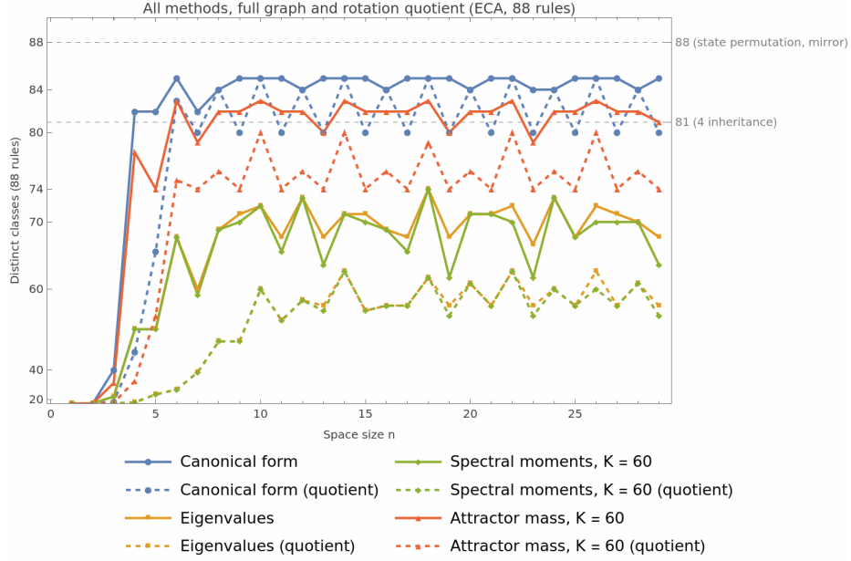
Fig. 8: Número de clases entre las 88 reglas representantes con cada método, en el grafo completo (línea continua) y en el grafo cociente (línea punteada), para n = 1, \dots, 29 . En los momentos se usa K = 60 , el valor que da más clases: al aumentar K el número de clases nunca disminuye.
