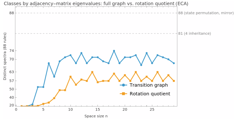
Fig. 4: Número de espectros distintos entre las 88 reglas representantes con el grafo de transición completo y con el grafo cociente por traslaciones, para n = 1, \dots, 29 (eje vertical en escala cúbica).
