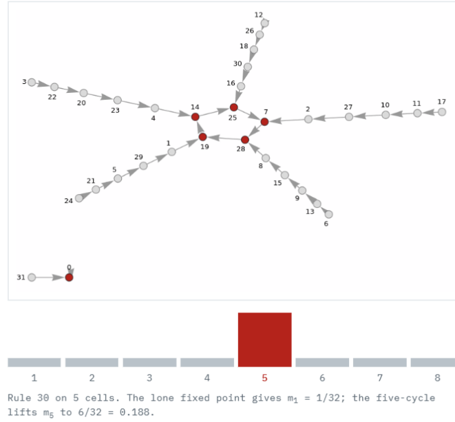
Fig. 6: Grafo de transición de la regla 30 con 5 células.
