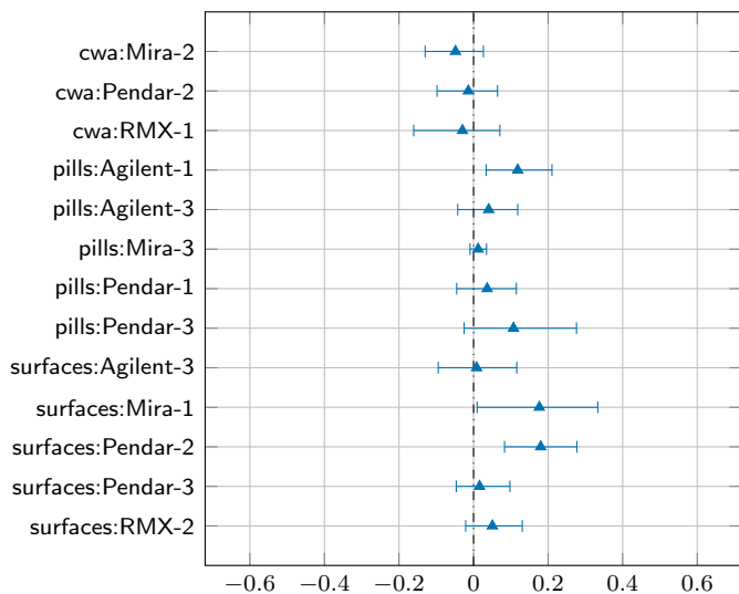
C. C-RANDOM-FOREST
