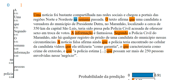
(d) Real classified as fake
