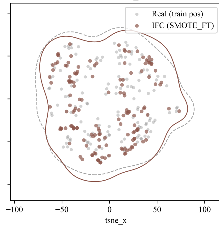
IFC (SMOTE_FT)
