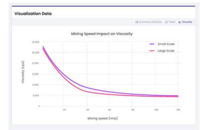
图为AI模拟的小型和商业规模的乳液粘度
