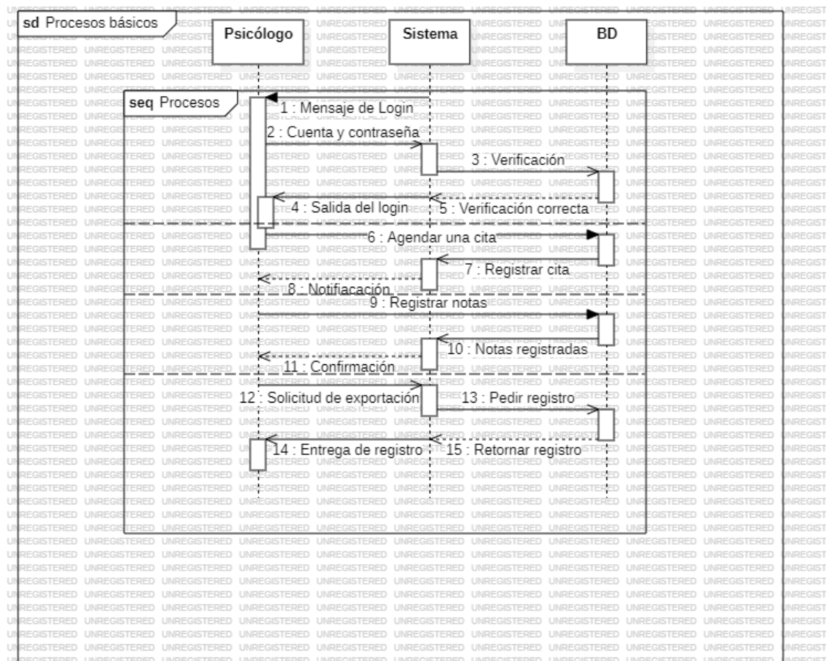
Ilustración 9. Diagrama de secuencias
