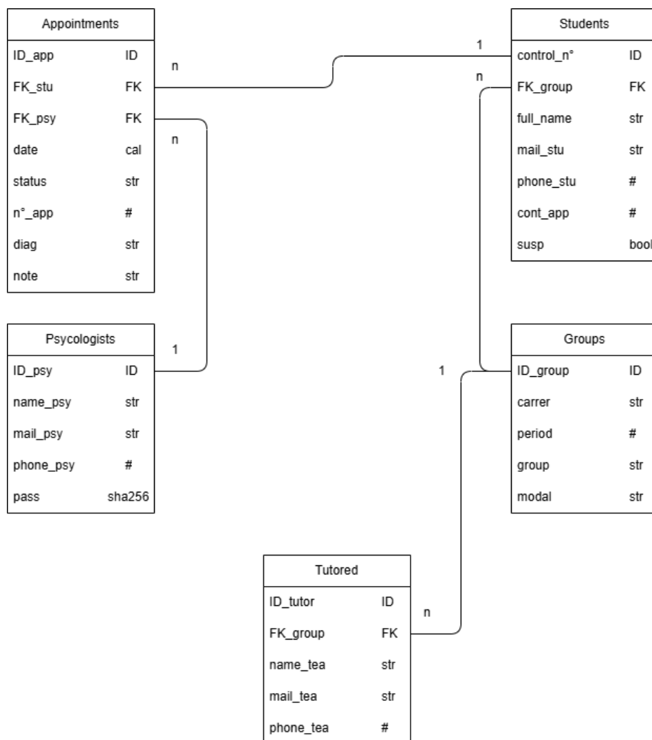
Ilustración 10. Modelo lógico-relacional del proyecto
