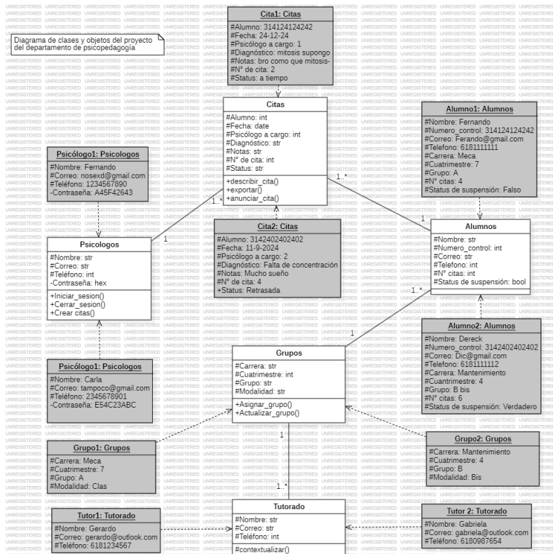
Ilustración 8. Diagrama de clases y objetos del programa
