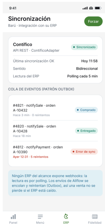
Figura 14: Proveedor — Estado de sincronización con el ERP
