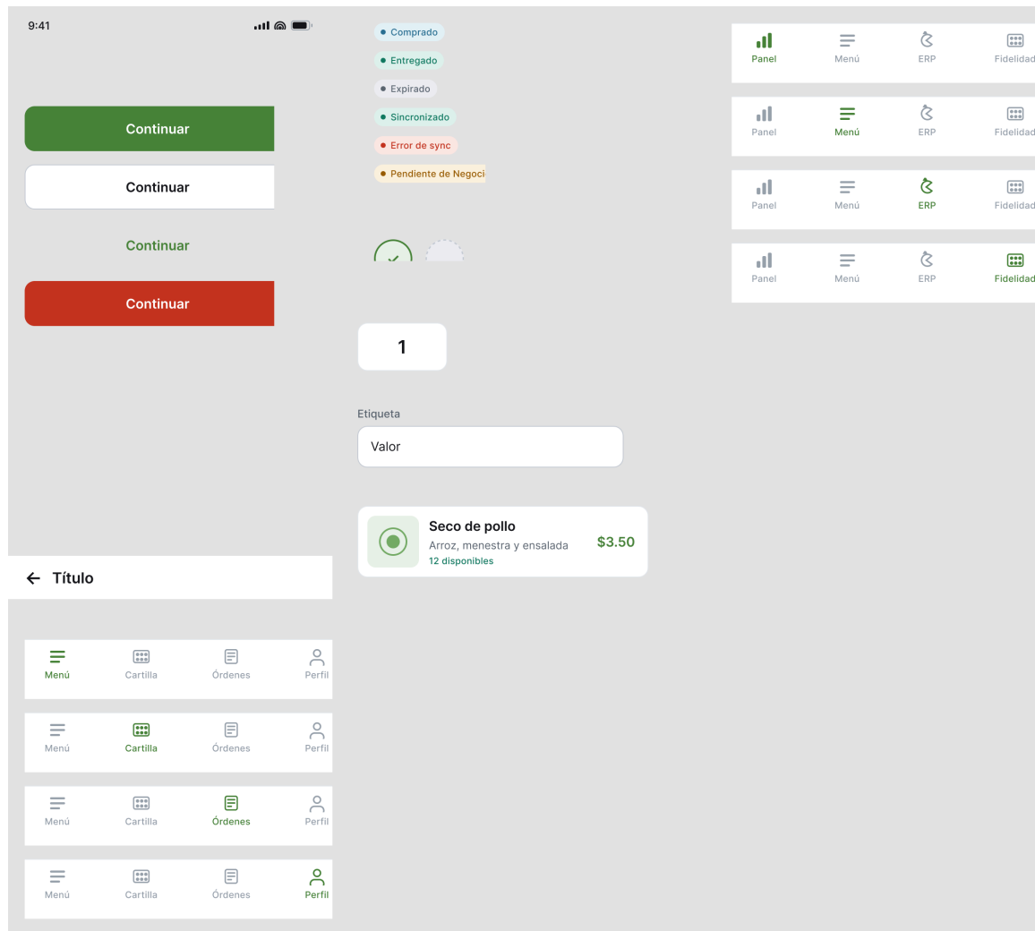
Figura 1: Sistema de diseño: variables, estilos de texto y componentes
