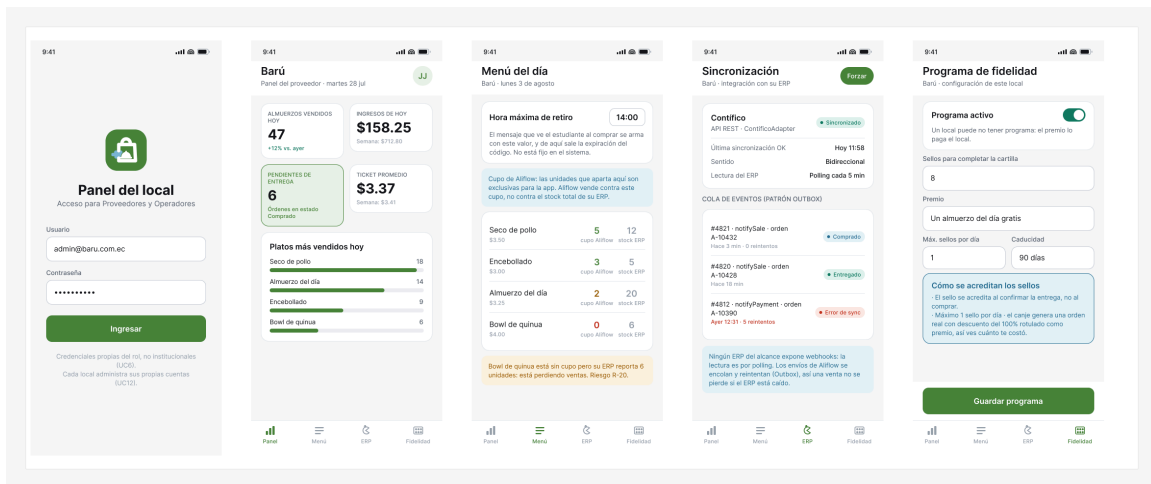
Figura 2: Flujo de ventanas del rol Proveedor
