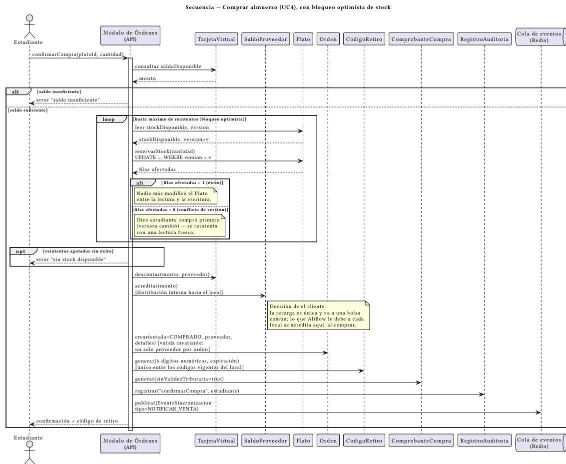
Figure 1: Secuencia: comprar almuerzo
