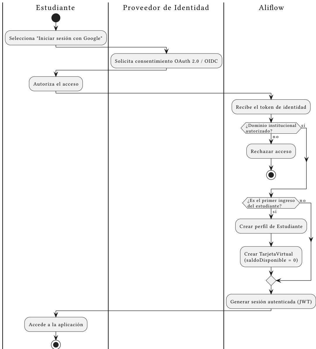
Figura 1: Actividad: autenticación
