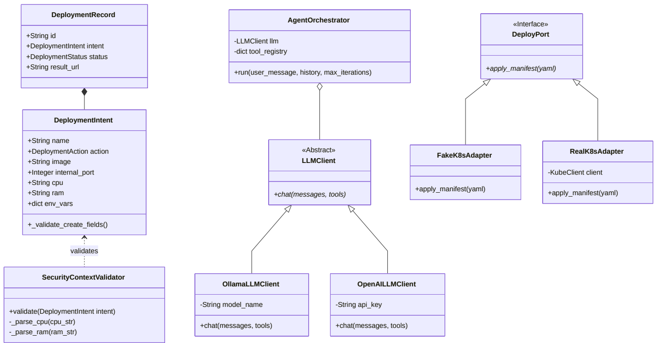
Figura 5: Diagrama de Clases (UML) resumiendo las principales entidades y contratos del núcleo lógico, destacando el uso del polimorfismo para la inyección de dependencias (LLMClient, DeployPort).
