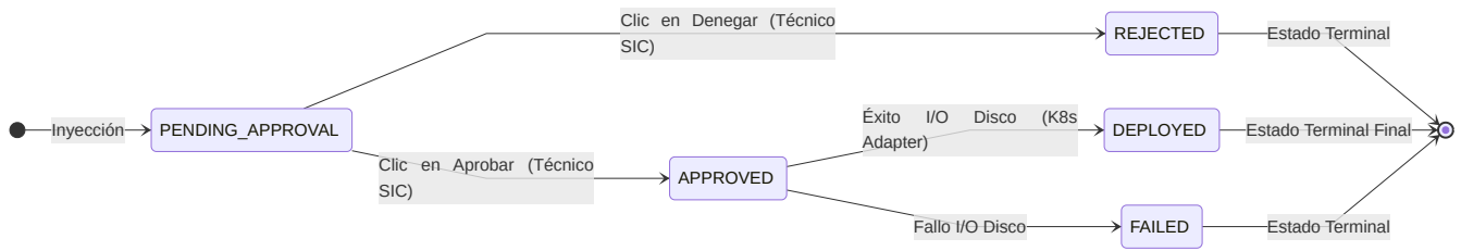
Figura 13: Grafo Dirigido Acíclico (DAG) que rige la Máquina de Estados Finita (FSM) del sistema.
