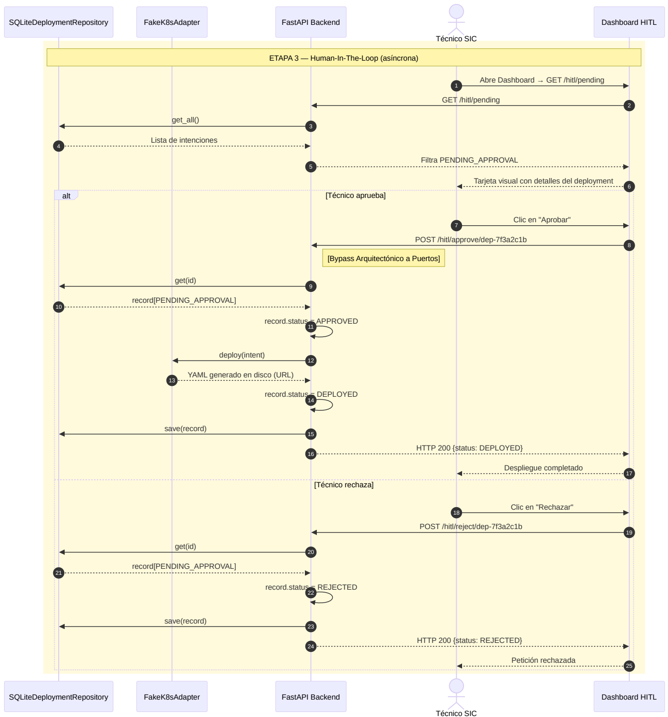
Figura 10: Diagrama de Secuencia E2E (Etapa 3). Decisión asíncrona del técnico humano, separando la inferencia de la ejecución.
