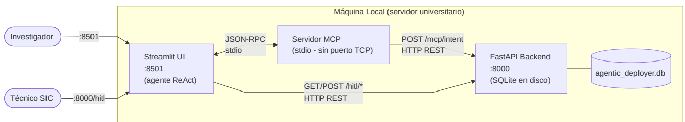
Figura 4: Diagrama de despliegue a nivel de proceso. Los cuatro componentes coexisten en la misma máquina; el servidor MCP se comunica por stdio sin exponer ningún puerto TCP.
