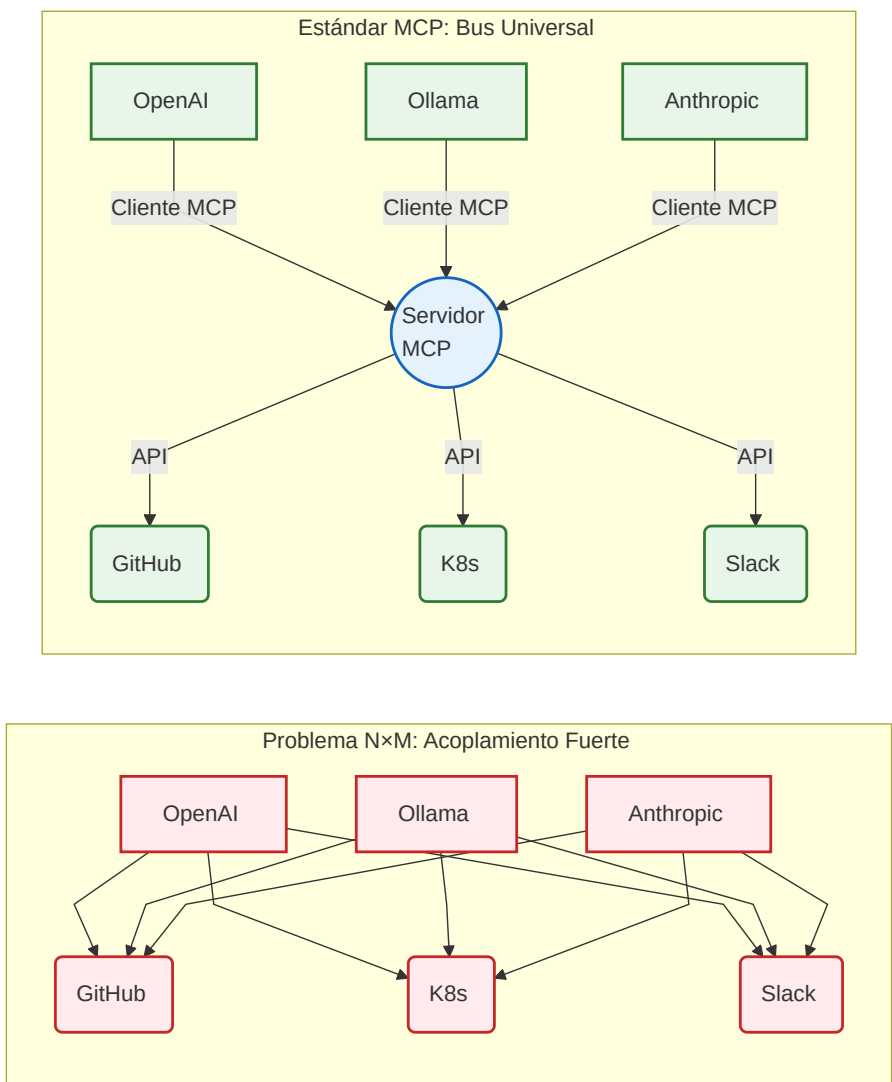
Figura 1: Contraste arquitectónico entre el problema de integración N×M (acoplamiento propietario) y la topología de Bus Universal propuesta por el protocolo MCP.
