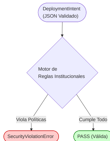
Figura 7: Visión general simplificada del SecurityContextValidator . Una rama de rechazo lanza el error para que ReAct se auto-corrija.
