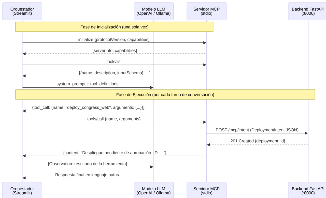
Figura 11: Ciclo de vida completo de un mensaje MCP. El protocolo JSON-RPC define tres fases: inicialización (handshake y descubrimiento de herramientas), ejecución (invocación y respuesta) y observación (retroalimentación al LLM).
