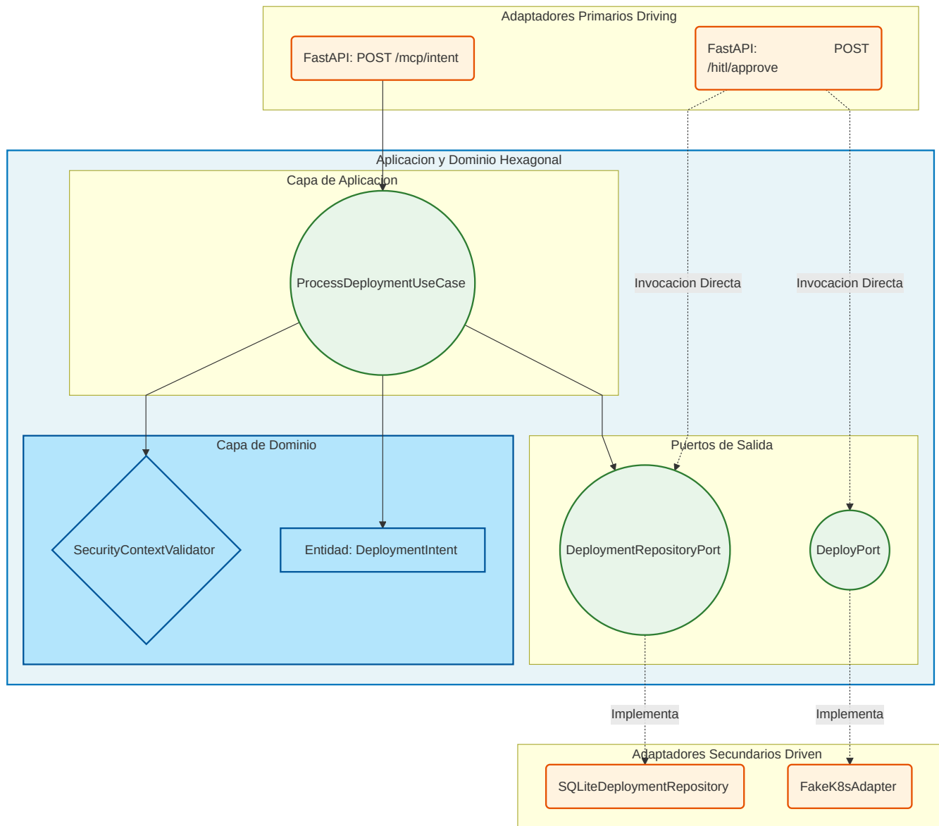
Figura 6: Topología de la Arquitectura Hexagonal. El flujo de control penetra desde los Adaptadores Primarios, pero la dependencia de código siempre fluye hacia el centro (Regla de Dependencia de Inversión).
