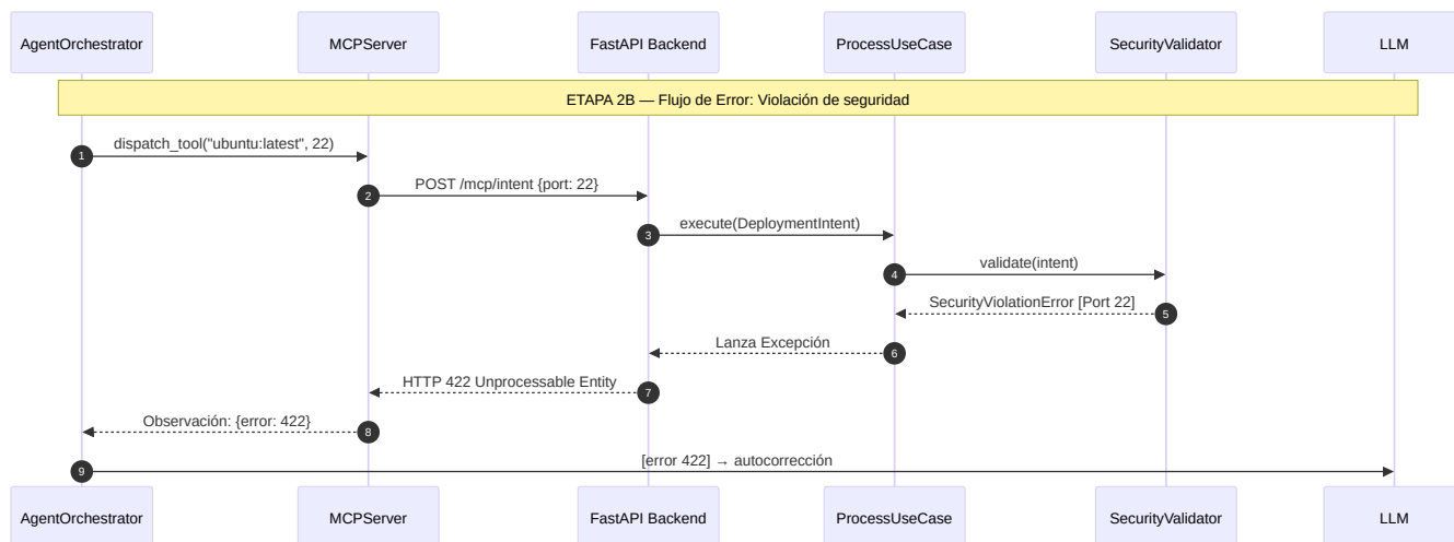
Figura 9: Diagrama de Secuencia E2E (Etapa 2). (Arriba) Camino feliz. (Abajo) Camino de error y autocorrección.
