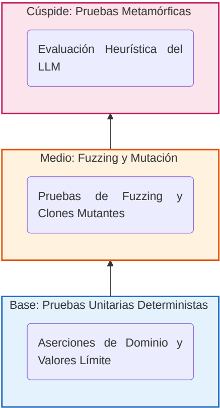
Figura 15: Arquitectura de la Pirámide Híbrida de Testing implementada en el Agentic Deployer , adaptando el modelo clásico a las exigencias de la Inteligencia Artificial Generativa.
