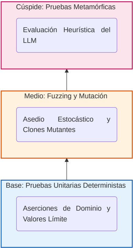
Figura 14: Arquitectura de la Pirámide Híbrida de Testing implementada en el Agentic Deployer , adaptando el modelo clásico a las exigencias de la Inteligencia Artificial Generativa.
