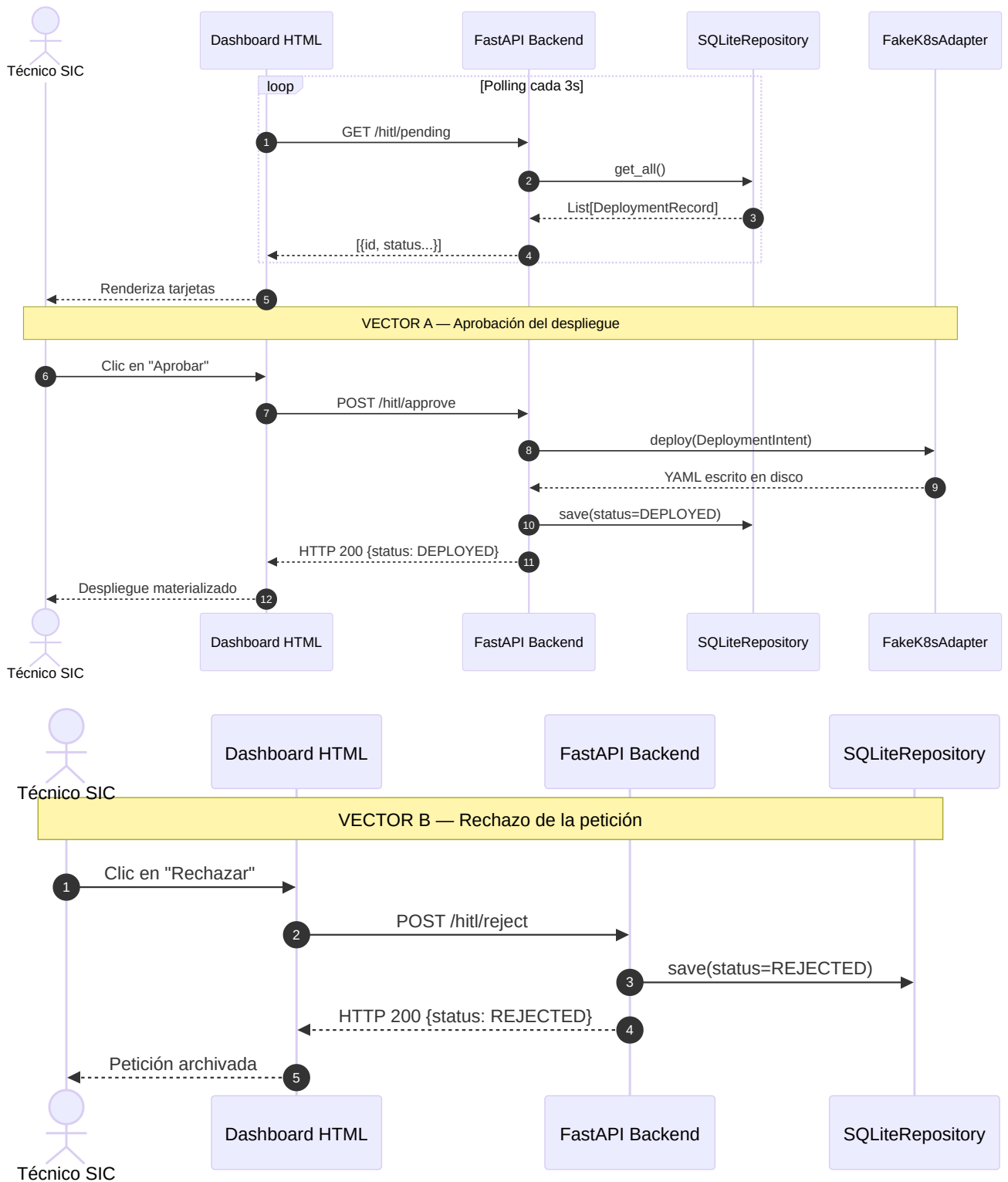
Figura 13: Diagrama de Secuencia del flujo HITL. (Arriba) Polling asíncrono y Vector de Aprobación. (Abajo) Vector de Rechazo (estado inmutable terminal).
