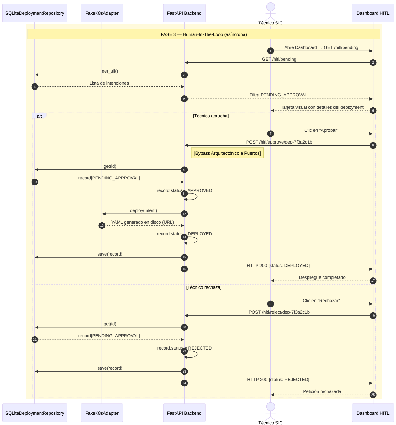
Figura 10: Diagrama de Secuencia E2E (Fase 3). Decisión asíncrona del técnico humano, separando la inferencia de la ejecución.
