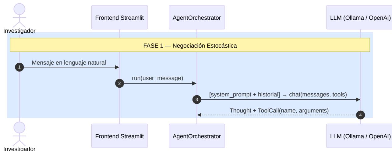
Figura 8: Diagrama de Secuencia E2E (Fase 1). Negociación cognitiva entre el Investigador y el LLM hasta alcanzar una intención.
