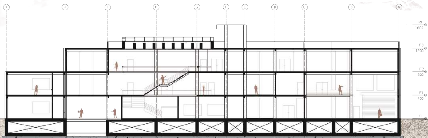
A-A Section
