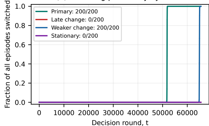
(d) Switching probability by round
