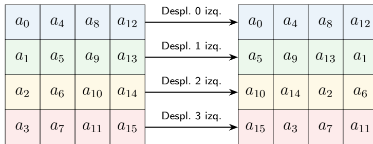
Figura 3.2: Algoritmo ShiftRows
