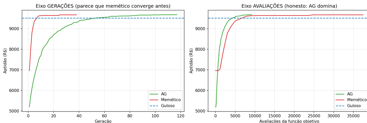
Figura 2 — Convergência por geração (esq., enganoso) vs. por avaliação (dir., justo).
