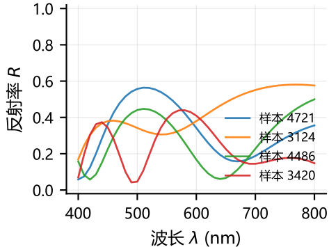
(C) TMM 生成的光谱 41 个波长点, 400–800 nm
