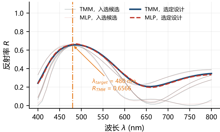
(A) 选定设计与五个入选候选
