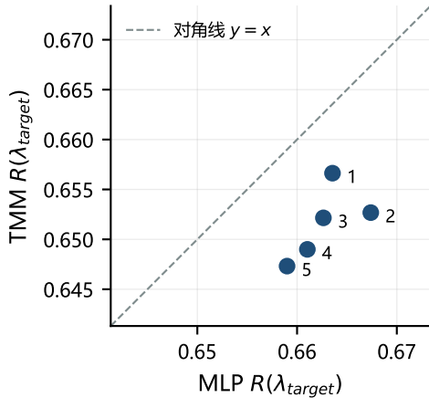
(B) MLP 排序经 TMM 验证
