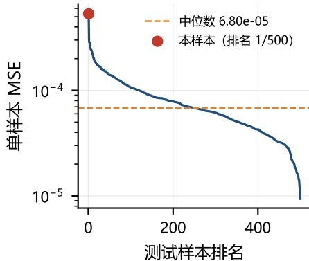
500 个测试样本的误差分布
