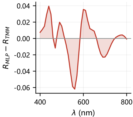
预测误差 \text{MSE} = 5.33\text{e-}04
