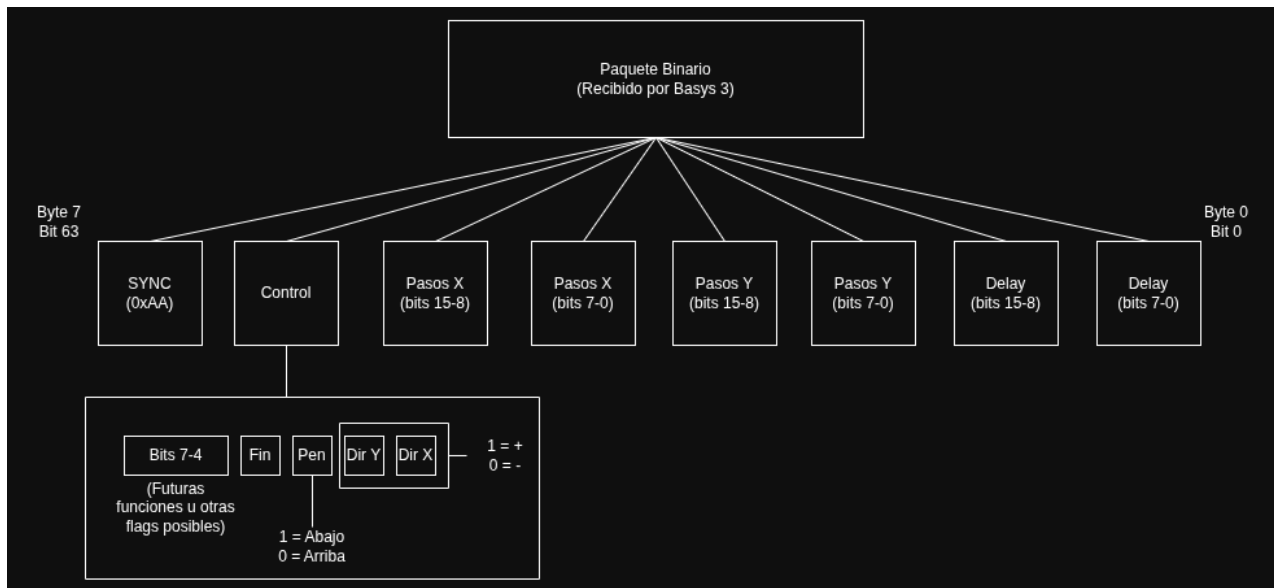
Figura 1: Paquete binario de instrucción G-code (fuente propia)
