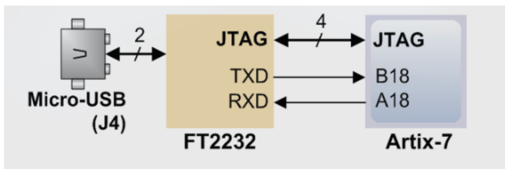
Figura 2: Puente UART Basys 3 [11]
